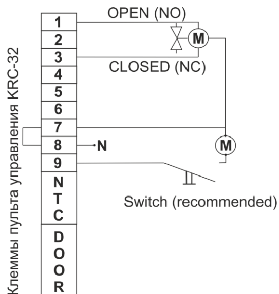
Рис.8. Электрическая схема присоединений привода регулирующего клапана и насоса для узла KVNB 6,3-20; KVNB 60-6,3-20; KVNB 21-20; KVNB 80-21-32 , с 2-х/3-х позиционным подключением.
