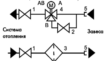
Рис. 1. Схема смесительного узла при \Delta P \geq 40 кПа с клапаном KVS KVNB 4,0-20; KVNB 6,3-20 и KVNB 6,3-20
